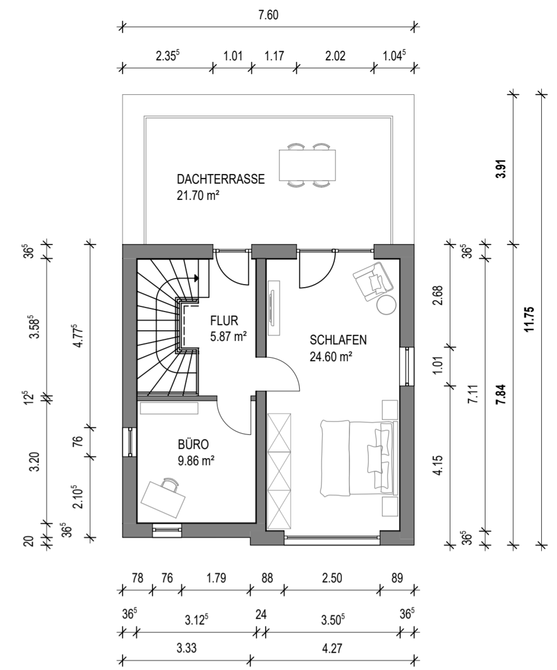
STAFFELGESCHOSS
