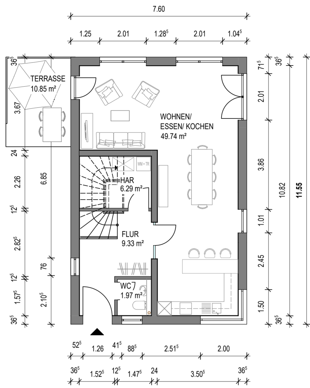
ERDGESCHOSS
