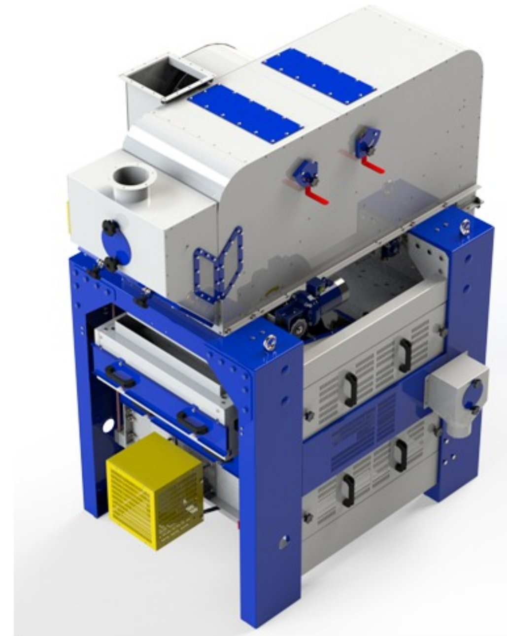
BISS mit Aspirationssystem und Sedimentationskammer
