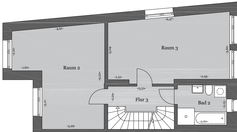
1.Obergeschoss
