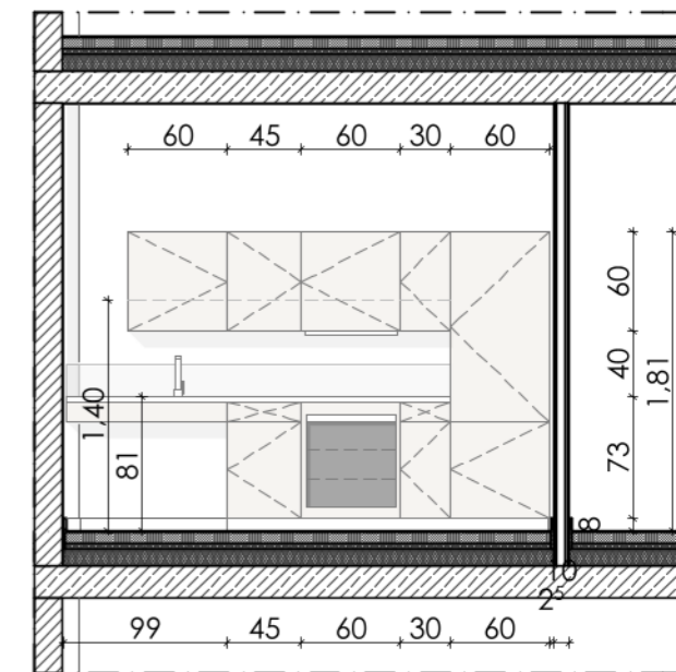
Variante rollstuhlgerechte Küchenzeile
