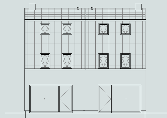
Hinteransicht
