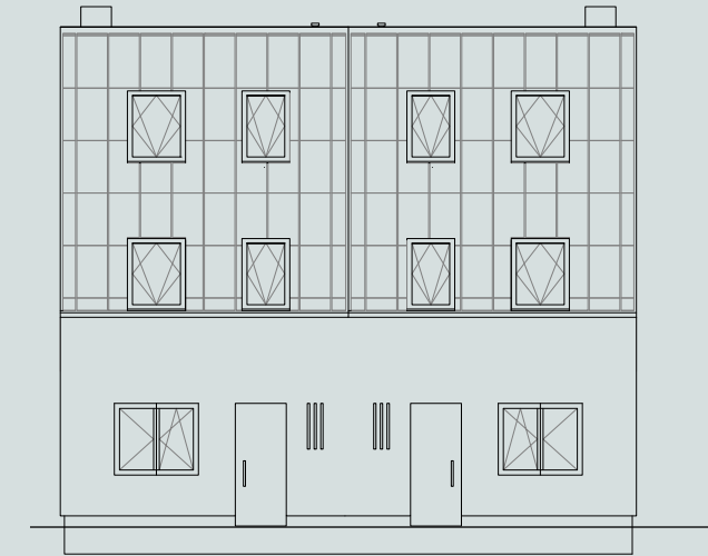
Frontansicht
