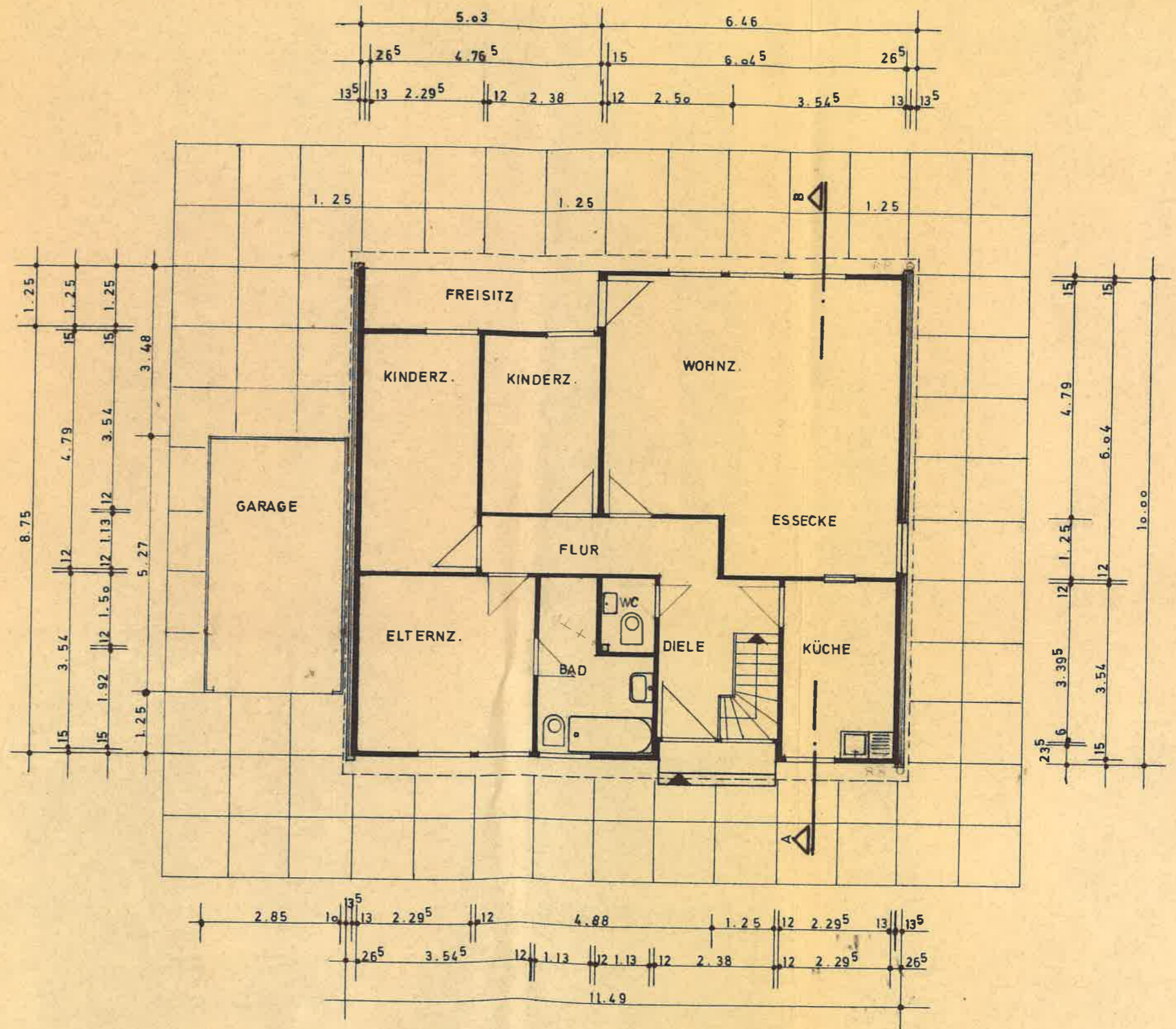
GRUNDRISS ERDGESCHOSS
