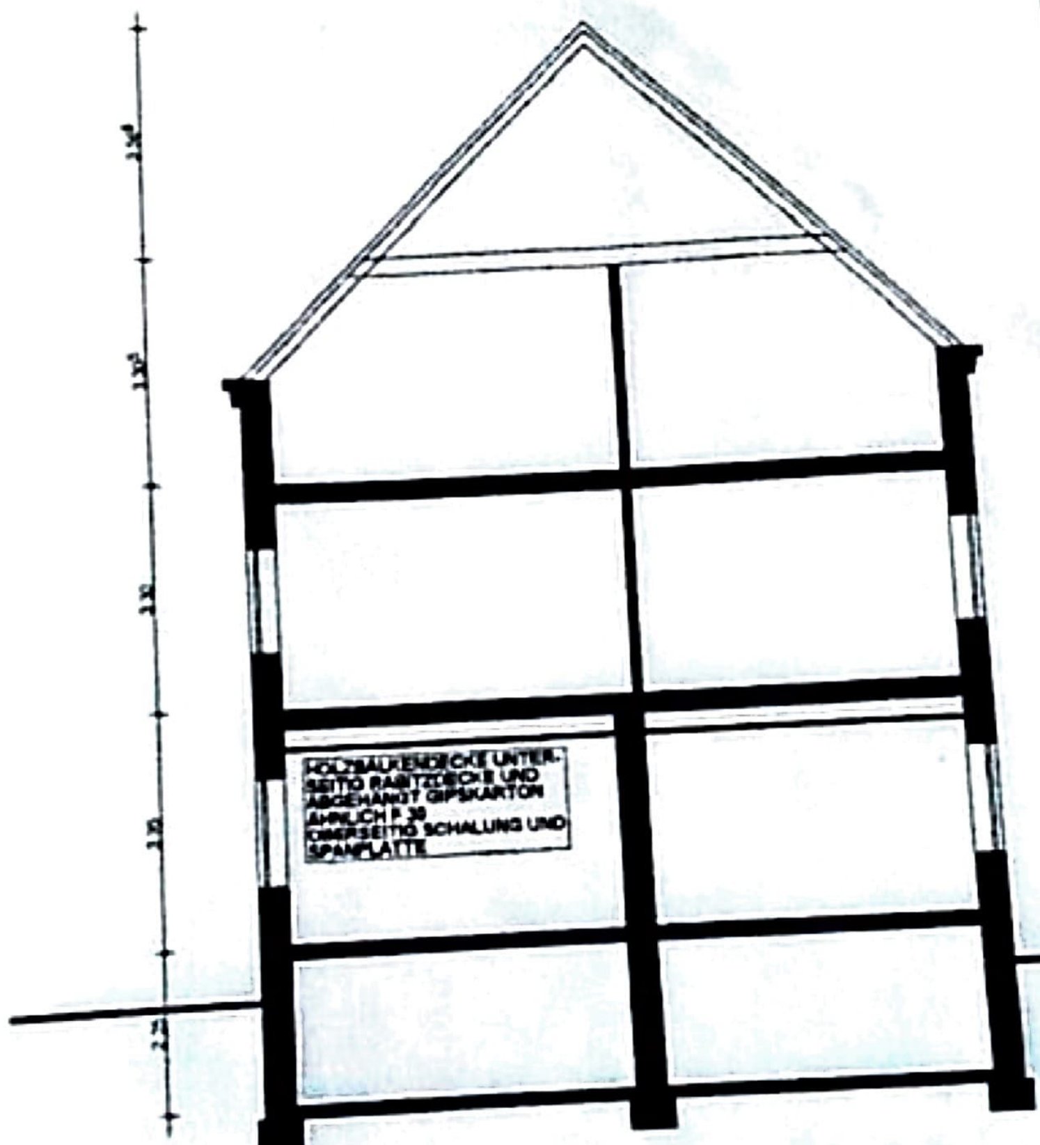
SCHNITT
