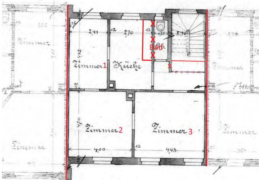
Grundriss 2. OG ohne Maszstab
