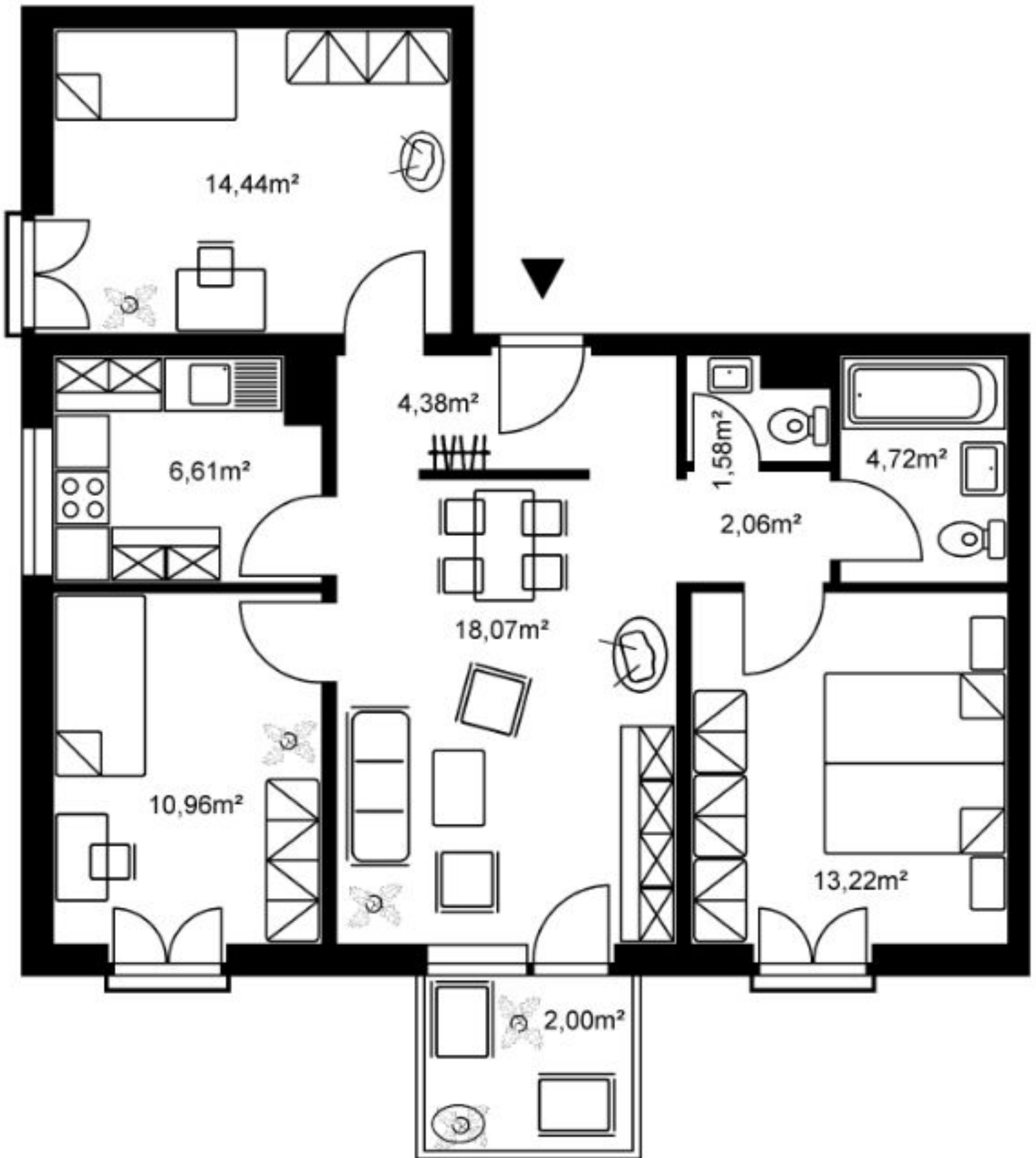
0 1 2 3 4 5 m Beispielmöblierung; Angaben unverbindlich.
