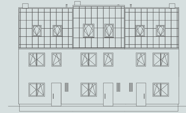
Frontansicht
