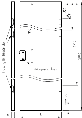
Türflügel ohne Falz
