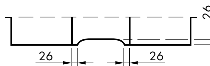
Unterschnitt in Vetro B Türflügeln
