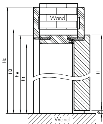
Vertikalschnitt OR
