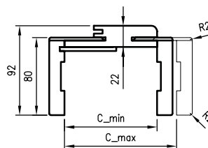
Schnitt ORB 095-300
