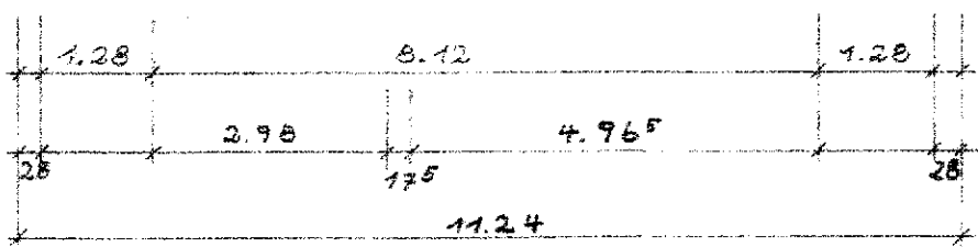
Dachgeschoss M. 1-100
