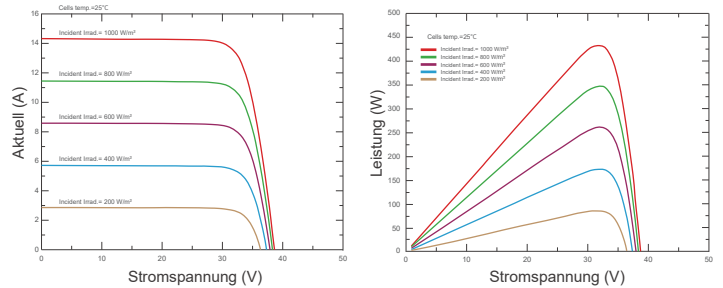
Strom-Spannungs- und Leistungs-Spannungskurven (SKT430M10-108D3)
