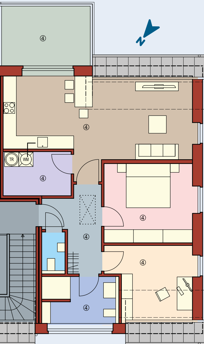
GRUNDRISS 1:100
