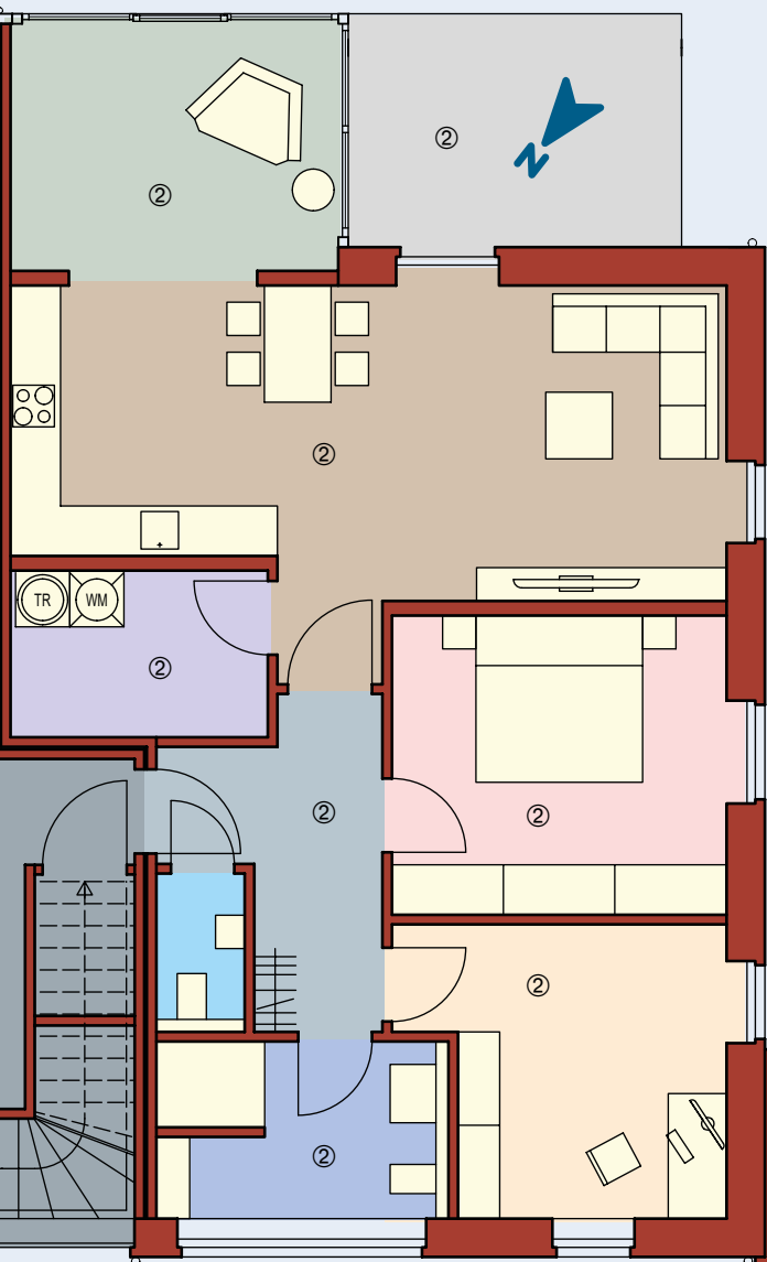
GRUNDRISS 1:100
