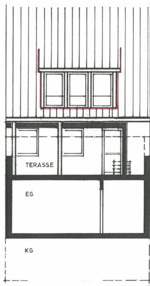
ANSICHT WEST
